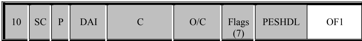
Optional PES Header
